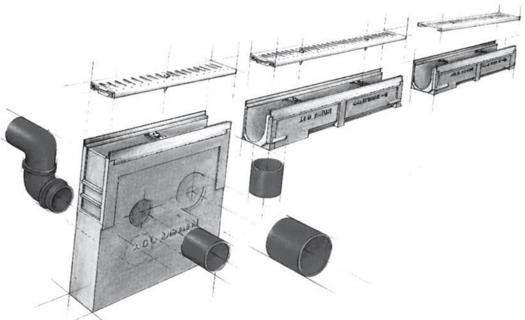
Overzicht ACO DRAIN® N 100 K met Quicklock®
